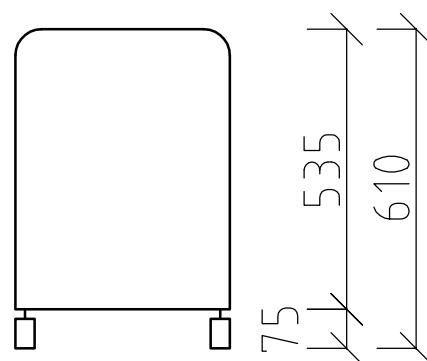
Bočný pohľad
