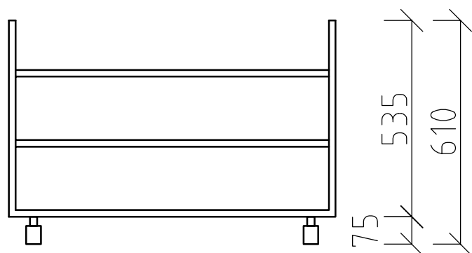
Pohľad
