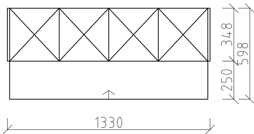
Pôdorys
