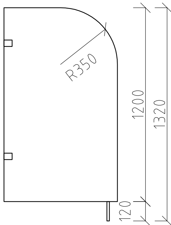
Pohľad
